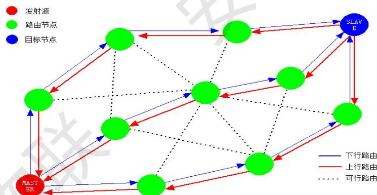
图 7.2.1 MESH 组网数据传递示意图
