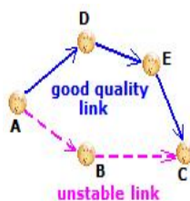
图 8.2 MESH 链路状态算法路由选择示意图
