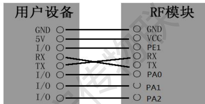
图 8.1 无线模块和用户设备连接示意图 (TTL)
