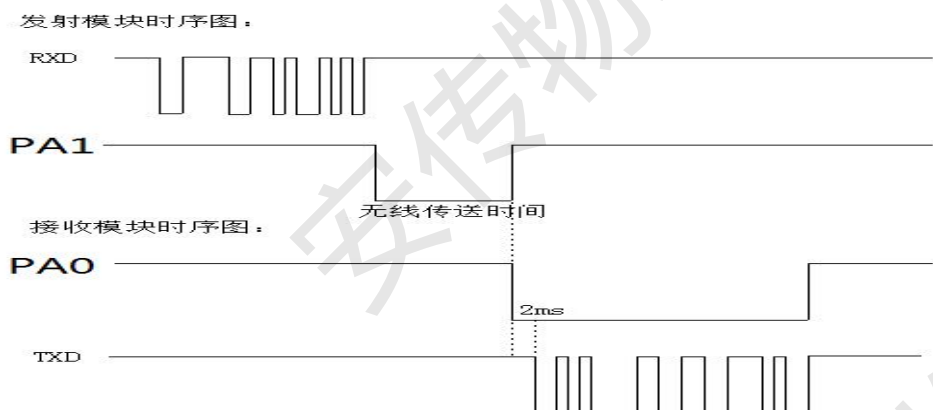
图10.1 透明模式下数据波形图
