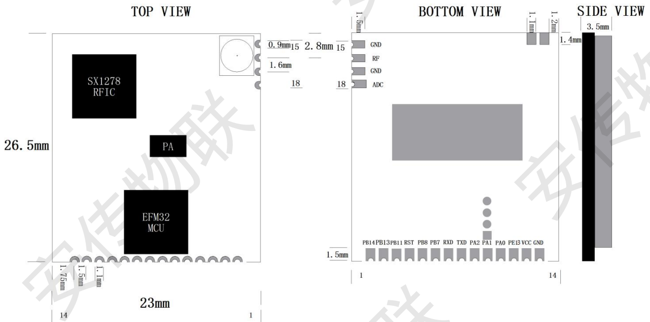
图 4.1 尺寸结构图
