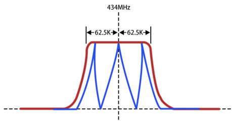
图 1 125K 扩频带宽图
