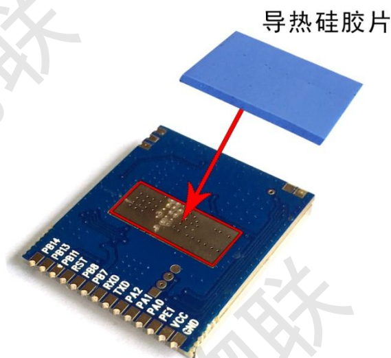
图 16.1 导热硅胶安装示意图
