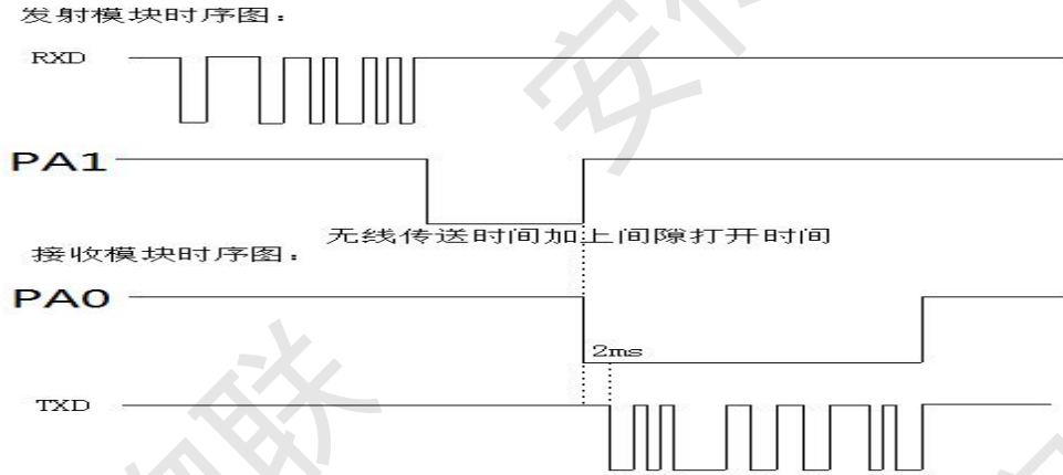
图10.3 节点模式下数据波形图
