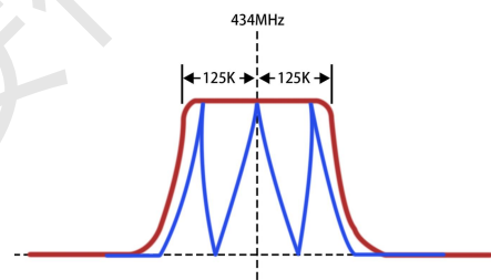
图 2 250K 扩频带宽图
