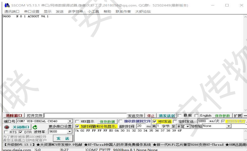
图 9. 3. 1 用串口调试助手获取模块当前串口参数和软件版本号
