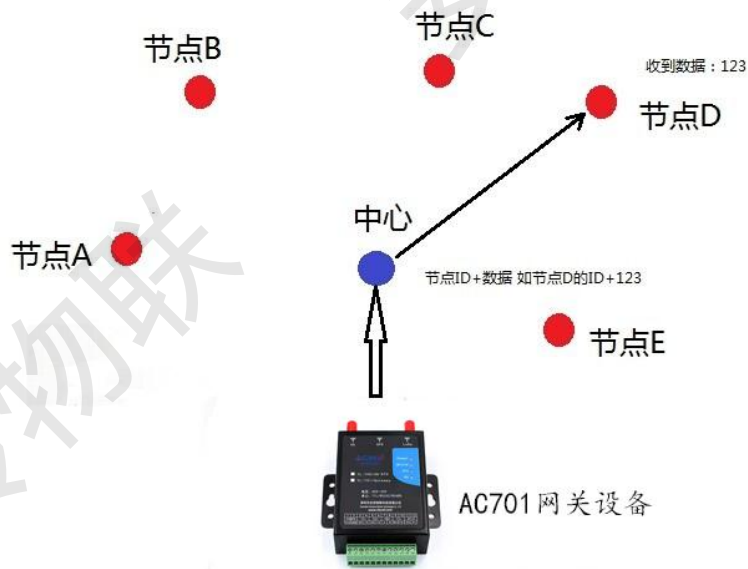
图 13.2 中心发数据到节点示意图
