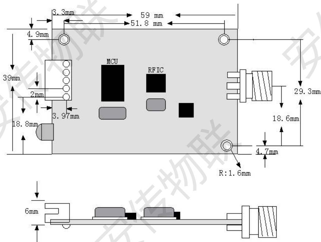
AC900IL尺寸示意图
