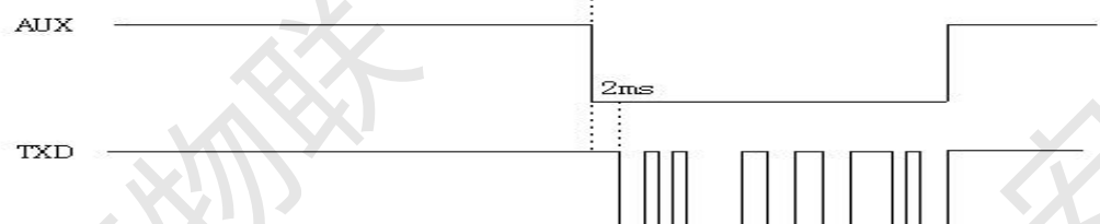
图9.2 低电流模式下数据波形图
