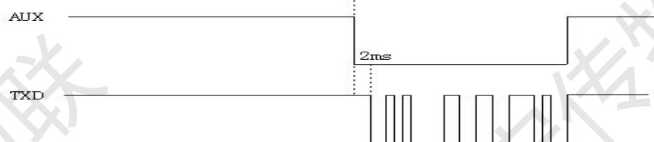
图9.1 全速模式下数据波形图
