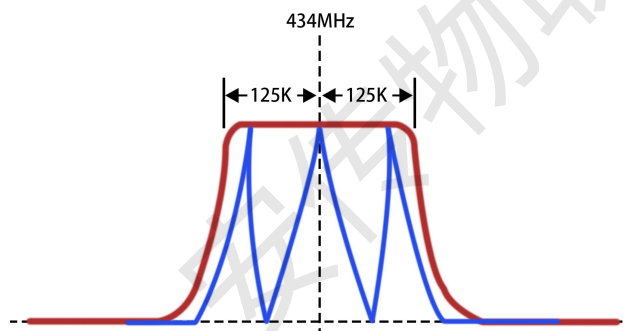
图 2 250K 扩频带宽图
